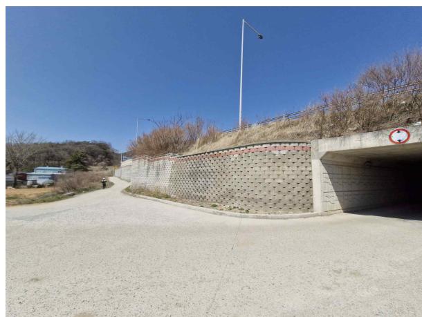
대산2교보강토옹벽 (STA.2+157.750~2+287.500(R))
