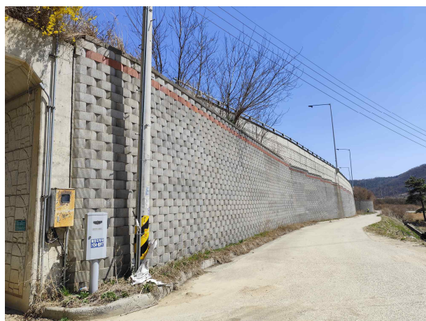
대산2교보강토옹벽 (STA.2+157.750~2+287.500(R))
